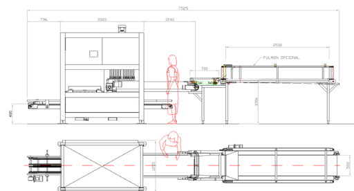
Vista en planta y alzado de Fompack Inline
