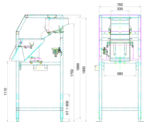
Vista en planta y alzado de tolva de pesado
