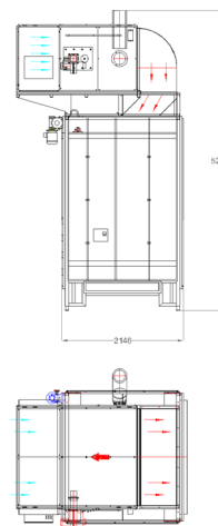
Vista en planta y alzado del túnel de secado vertical
