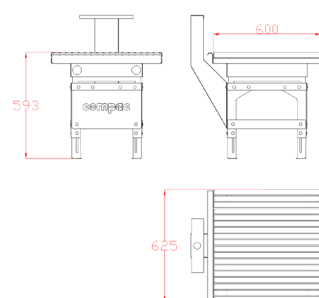
Vista en planta, corte y alzado de verificador de peso estándar.
