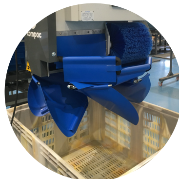
Cabezal con cepillos para fruta delicada en RF3
