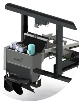
Esquema en 3D de llenadora de bins modelo "RF5"
