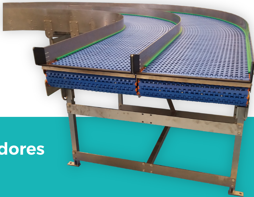
Transportador de banda modular
